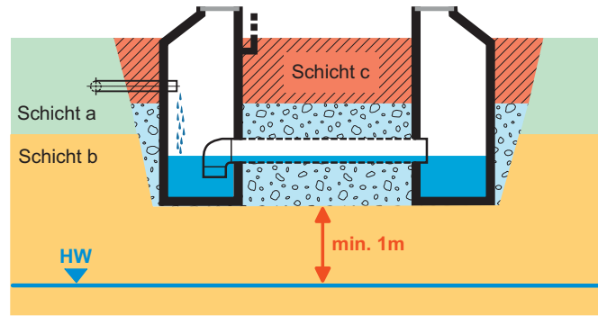
Typ 3: Versickerungsstrang
